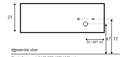
Aan- /afvoer PITCH Rechts 100 / 120 / 140 / 160 (designsifon laag model)
